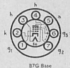
B7G Base
