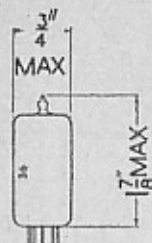
B7G Base
