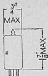
B7G Base
